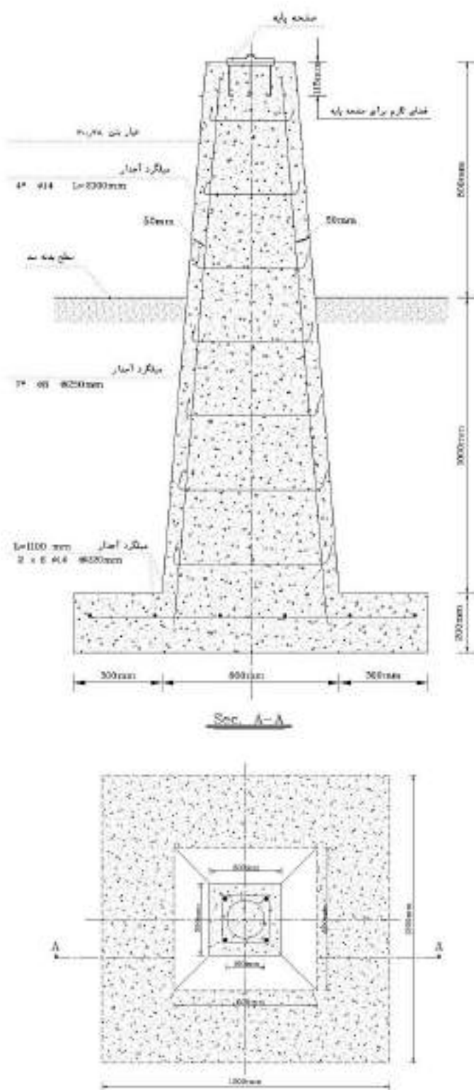
شکل ۱۳-۰ نقطه نشانه روی بدنه و تاج سدهای خاکی، مناطق زمین لغزش خاکی (در شبکه‌های کلاسیک)، برمه‌های نیروگاه‌ها
