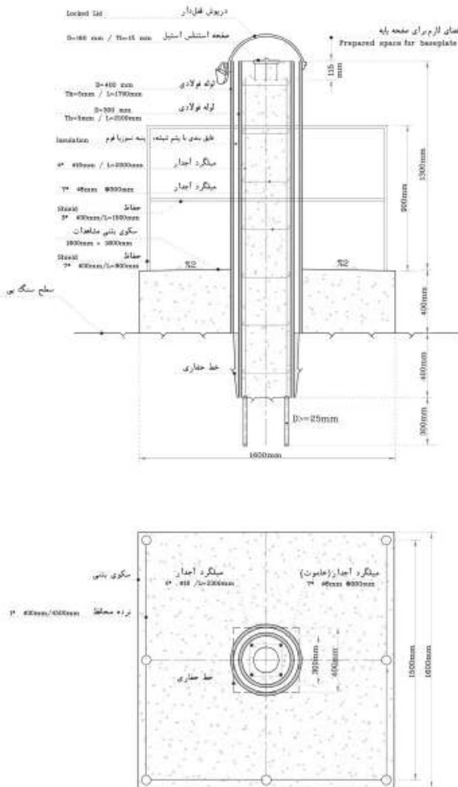
شکل ۳-۱ پیلار روی پی سنگی
