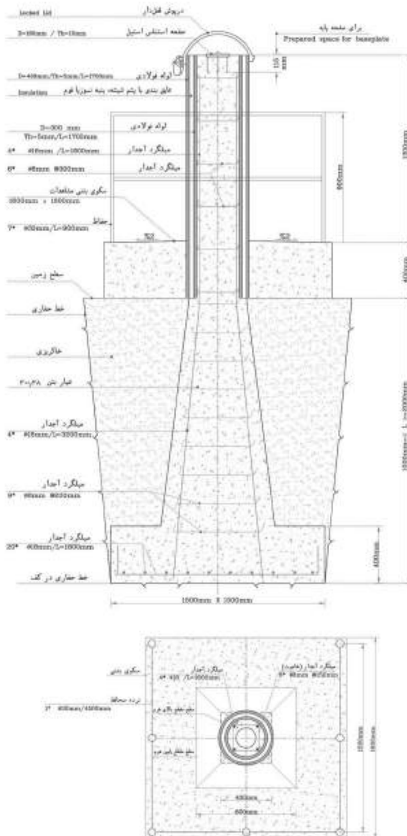
شکل ۳-۳ پیلار روی پی غیر سنگی یا روی تاج سد خاکی
