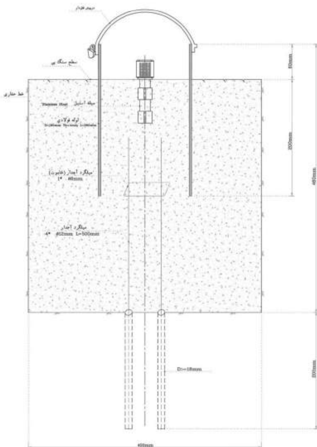
شکل ۴-۰ نقطه مبنای ارتفاعی روی پی سنگی
