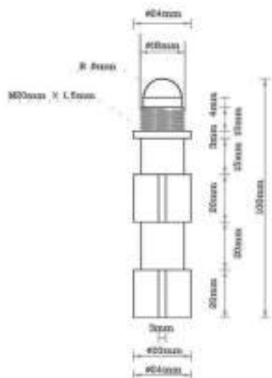
جنس میله : استیل ۳۱۶ قطر میله : ۲۴ میلیمتر
